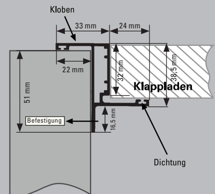
Einbauzarge (Nicht maßstabsgetreu)
