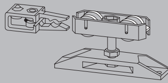
Zubehörkit manueller Schiebesatz
