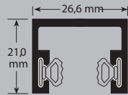
Führungsschiene unten mit Gleitkeder
