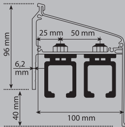
Profilkit 2-spurig
