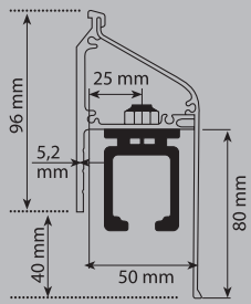
Profilkit 1-spurig
