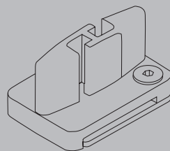
Gleiter mit Klemmplatte
